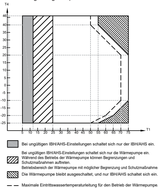
T1-Wasseraustrittstemperatur T4-Außenumgebungstemperatur
