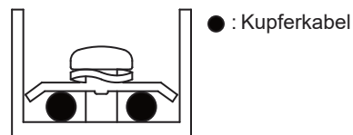
Korrekte Stromversorgungsverkabelung
