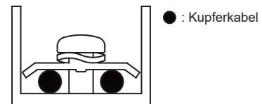
Korrekte Stromversorgungsverkabelung
